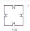
HB-037 10分方柱 10cm square column 氧化原色L5000mm, L6000mm
