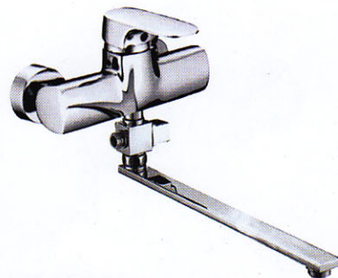
LB23131-F30 wall mounted kitchen mixer Ванна-душ, длинный излив
