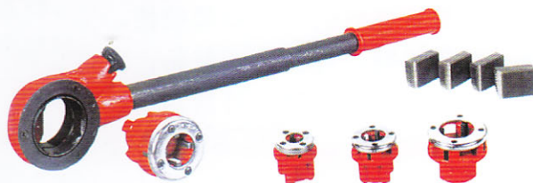
62 型管子铰板 RATCHET DIE STOCKS TYPE 62
