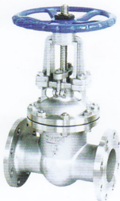
Z41W-16C 闸阀
